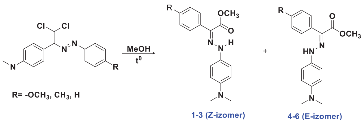
Scheme 3. Metil-2-(4-(dimetilamino)-fenil)-2-(2-(p-əvəzli)hidrazon)asetatların sintezi
