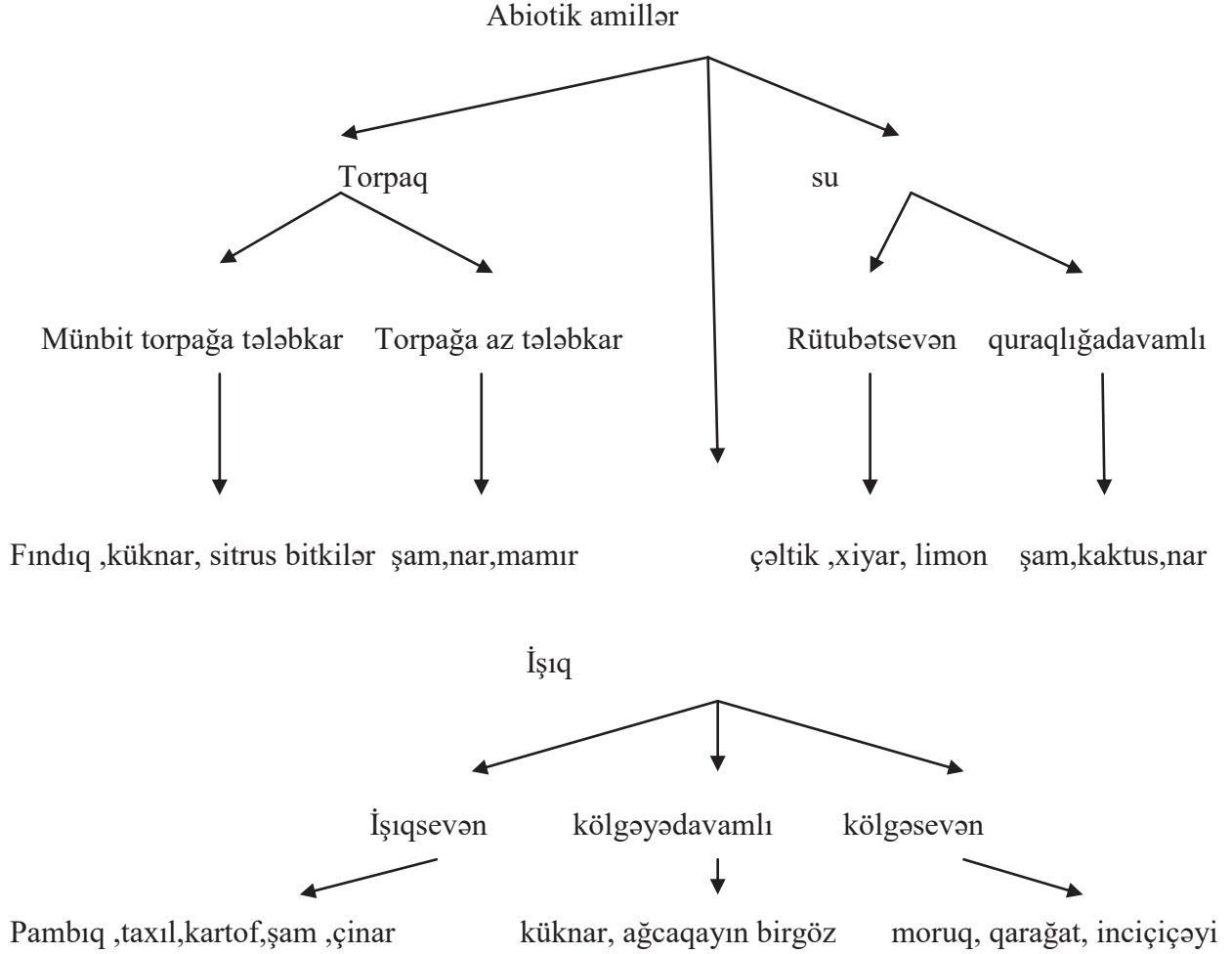
Sxem 2.
